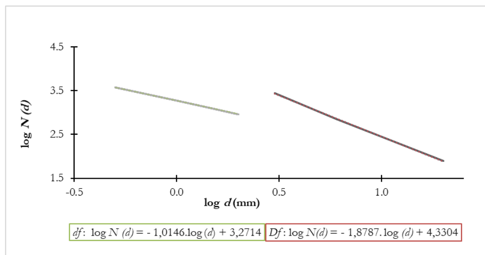
Figura 4. Gráfico log d x log N ( d ) para determinação de df e Df para a bacia do rio Faxinalzinho.
